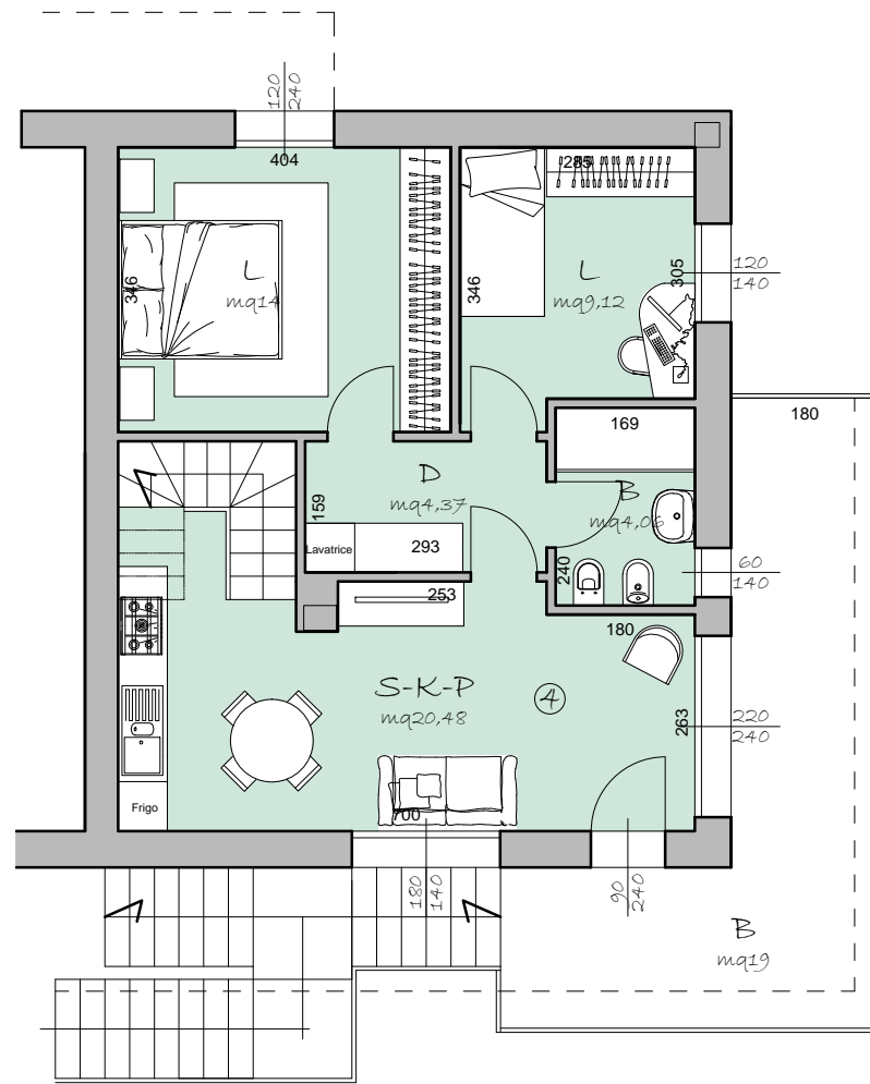
PIANO PRIMO scala 1:100
