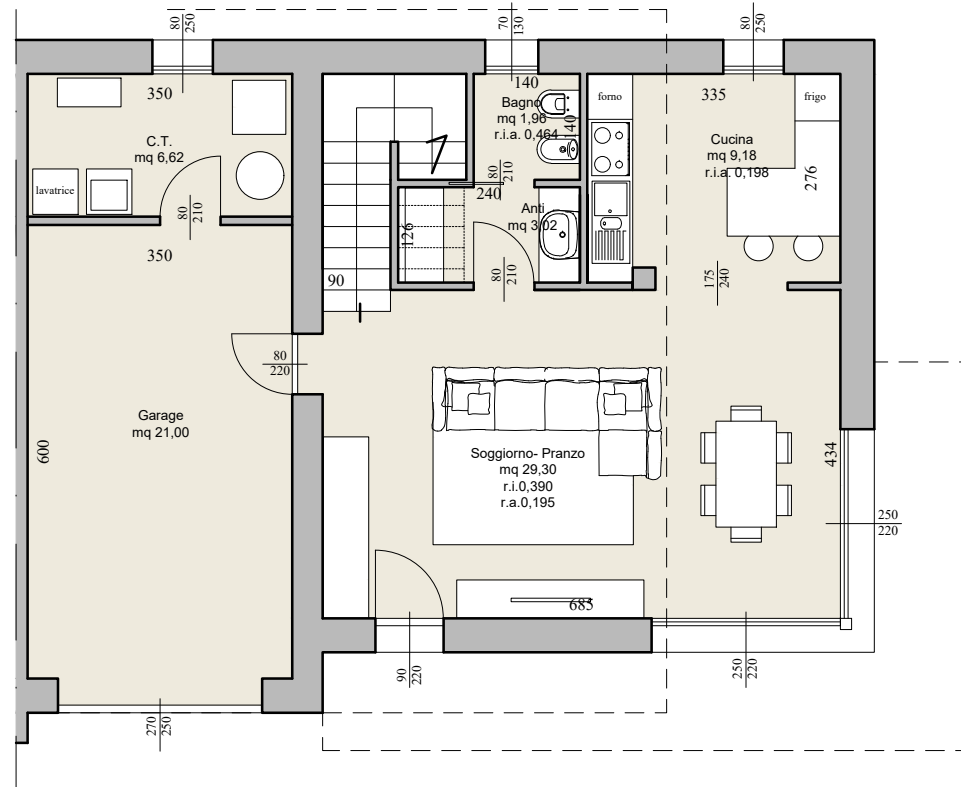
PIANTA PIANO TERRA sc 1:100
