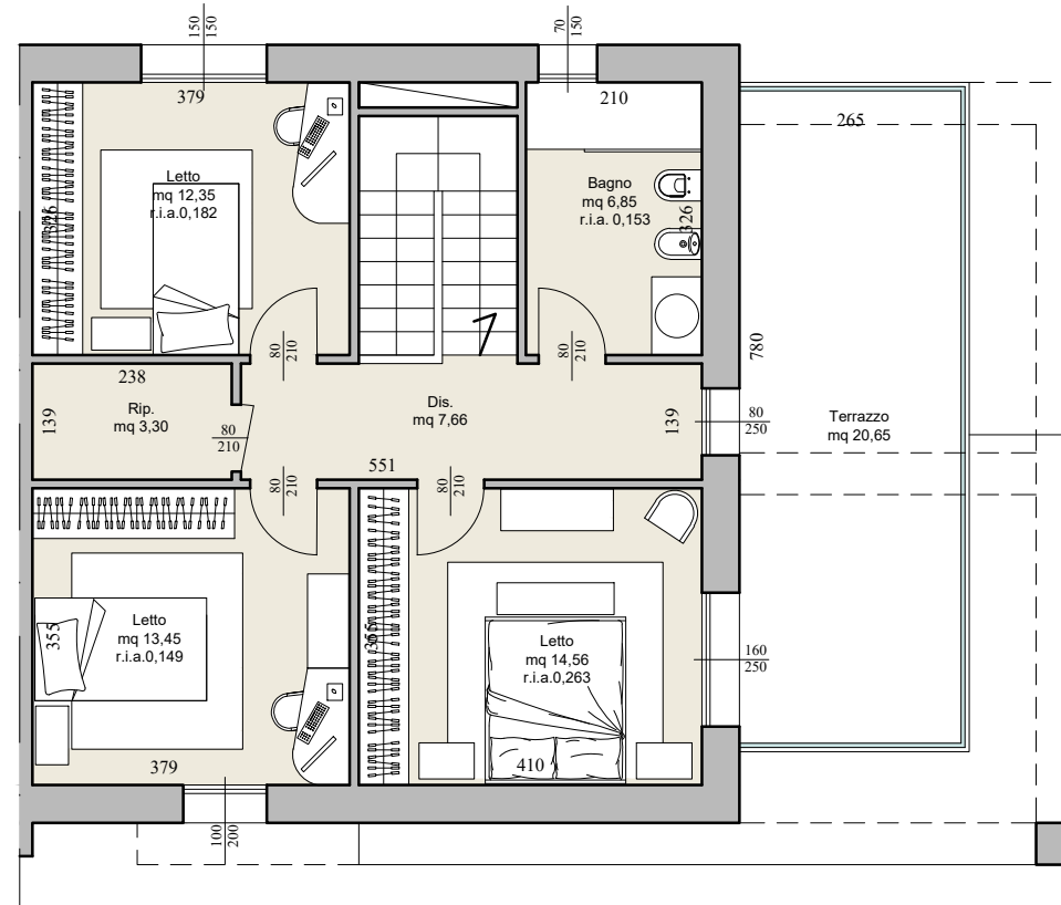
PIANTA PIANO PRIMO sc 1:100
